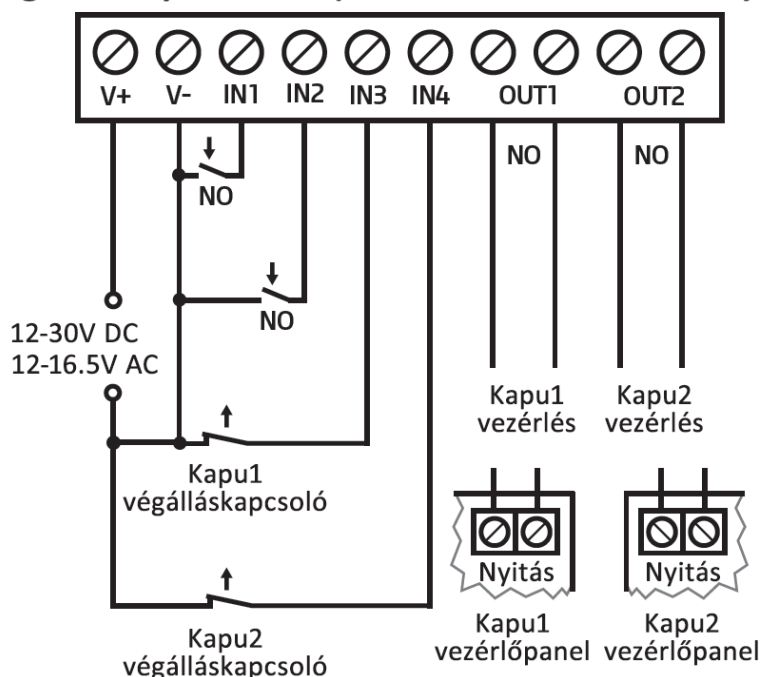
Egy vagy két kapu bekötése végálláskapcsolóval (1. és 2. vezérlési módok)
